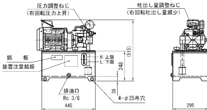
寸法表 (単位:mm)
