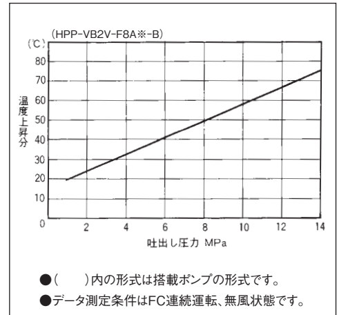
作動油の温度上昇早見表(油温=室温+温度上昇分)
